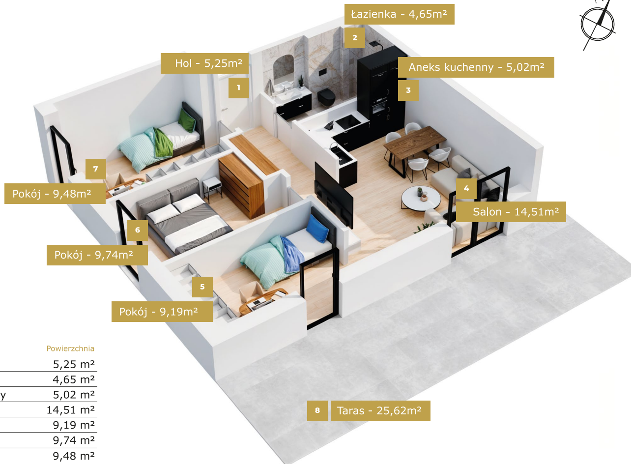
Rzut kondygnacji
