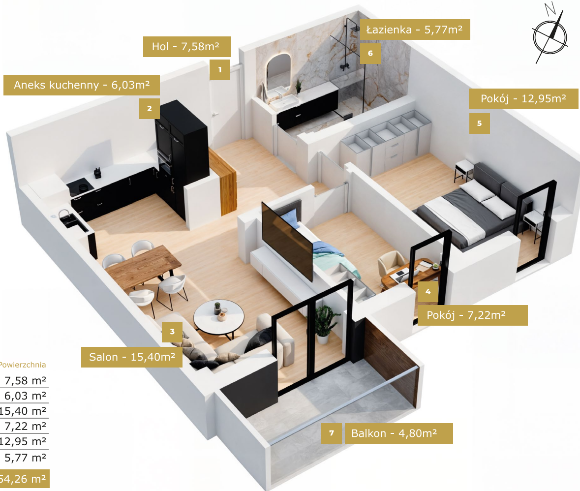
Rzut kondygnacji
