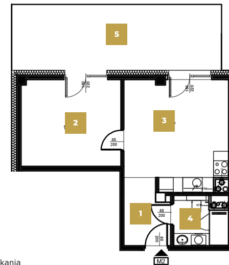
Rzut kondygnacji
