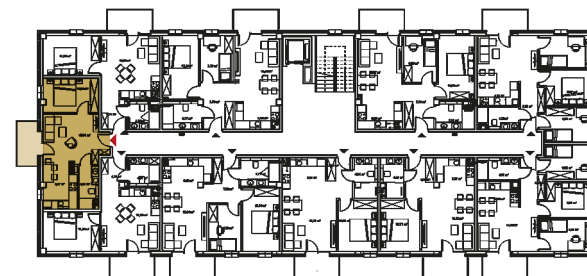
Rzut kondygnacji
