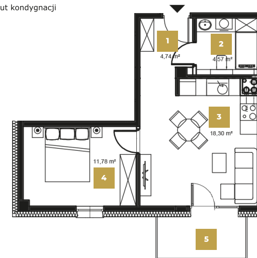
Rzut mieszkania
