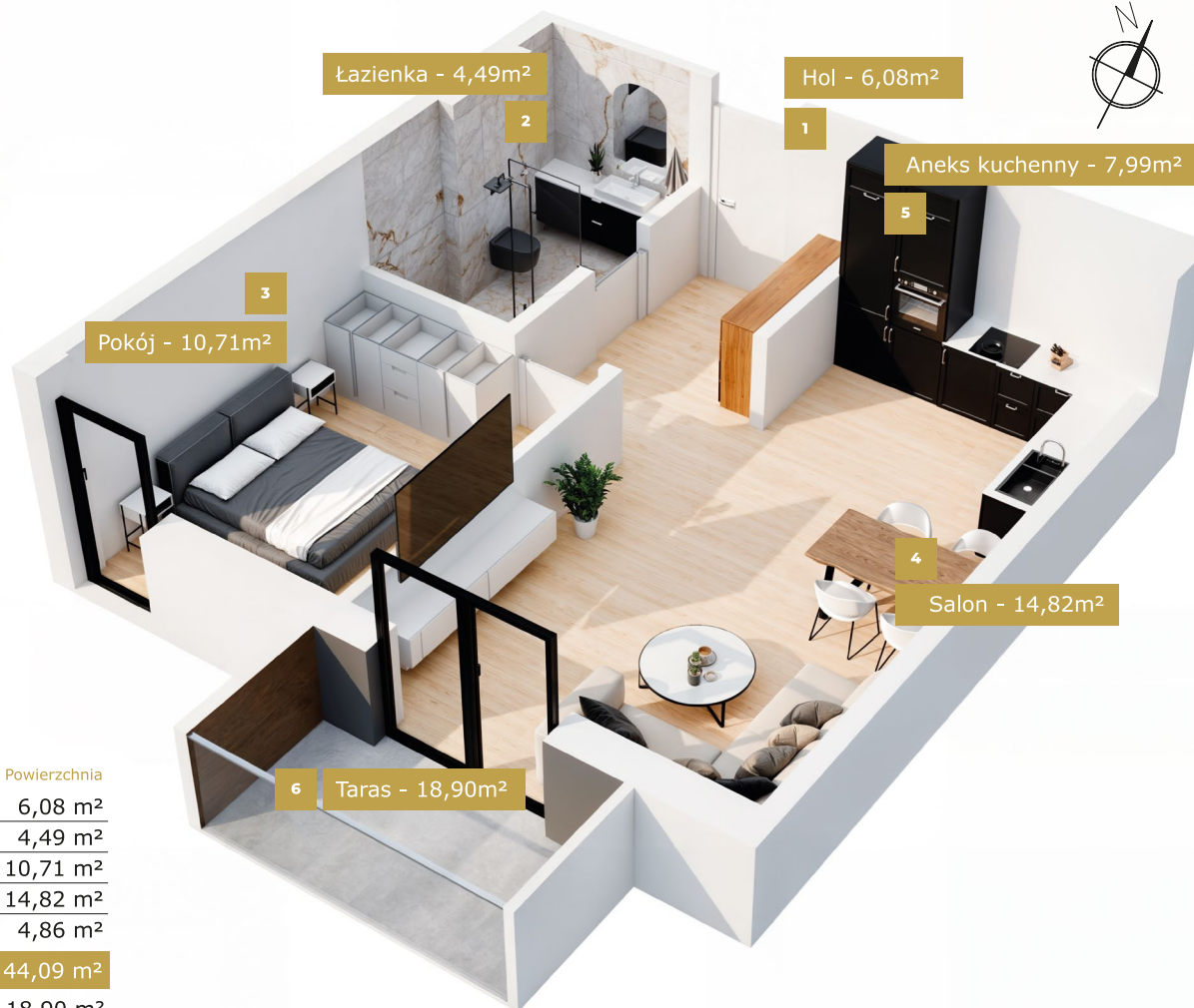
Rzut kondygnacji
