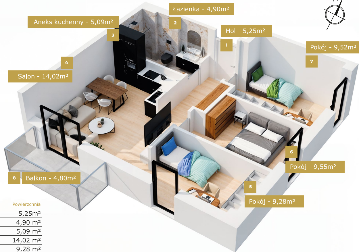
Rzut kondygnacji
