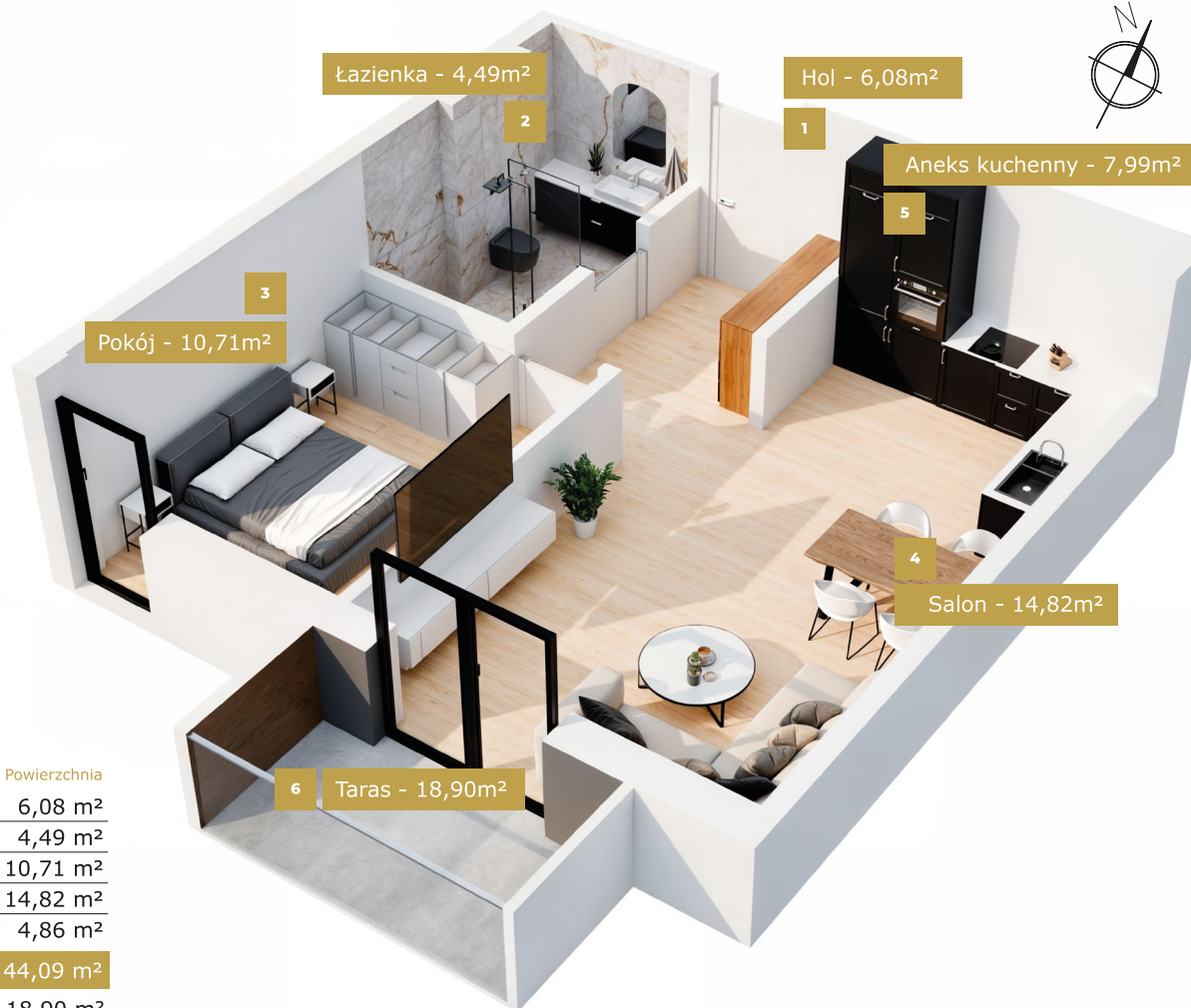
Rzut kondygnacji
