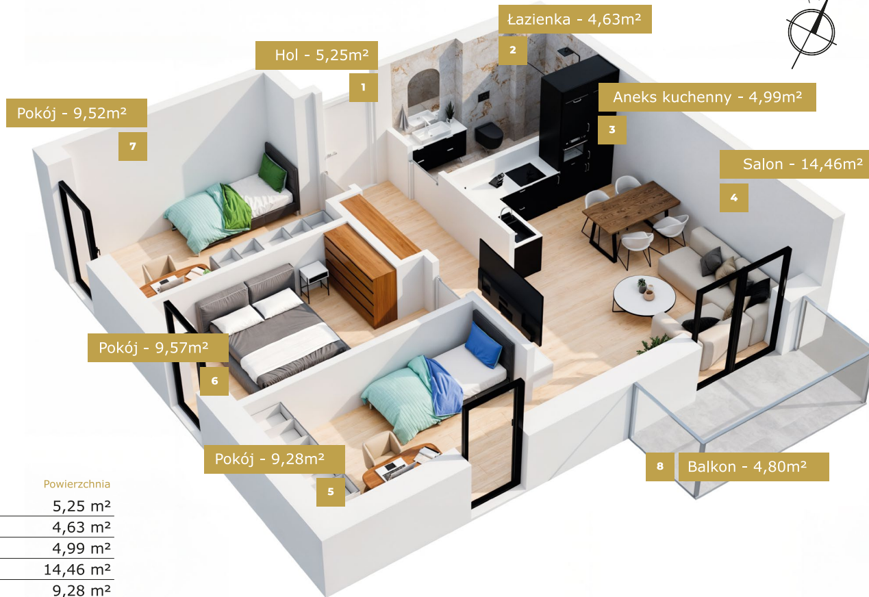
Rzut kondygnacji
