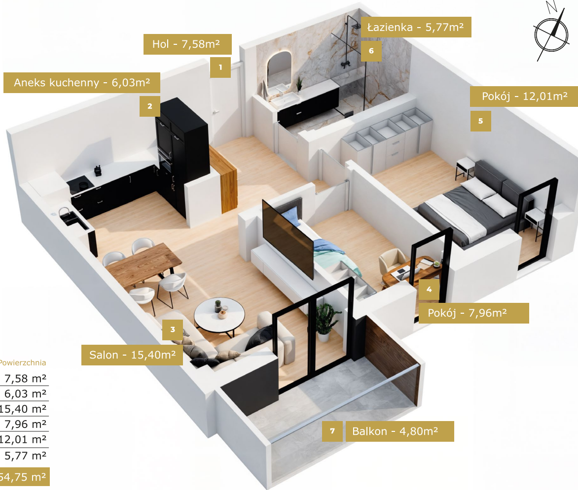
Rzut kondygnacji
