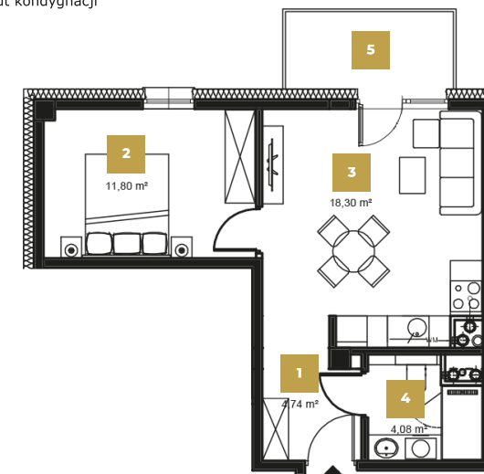
Rzut mieszkania
