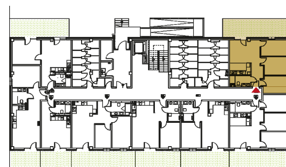
Rzut kondygnacji
