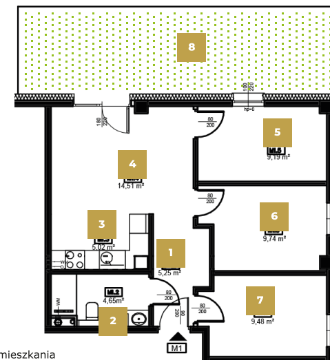
Rzut mieszkania
