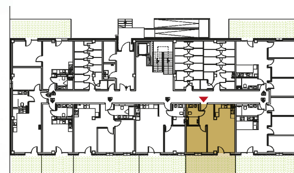
Rzut kondygnacji
