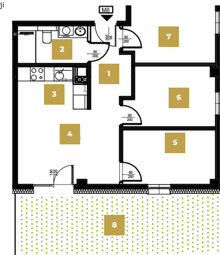
Rzut kondygnacji
